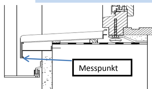
Z-Profil unter der Fensterbank
