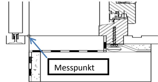
T-Profil im Boden eingelassen
