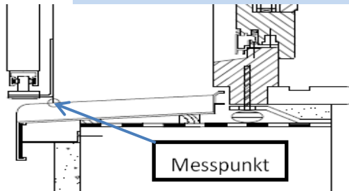
T-Profil über der Fensterbank
