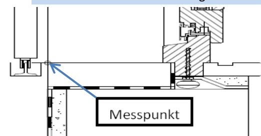
T-Profil auf dem Bodenbelag montiert
